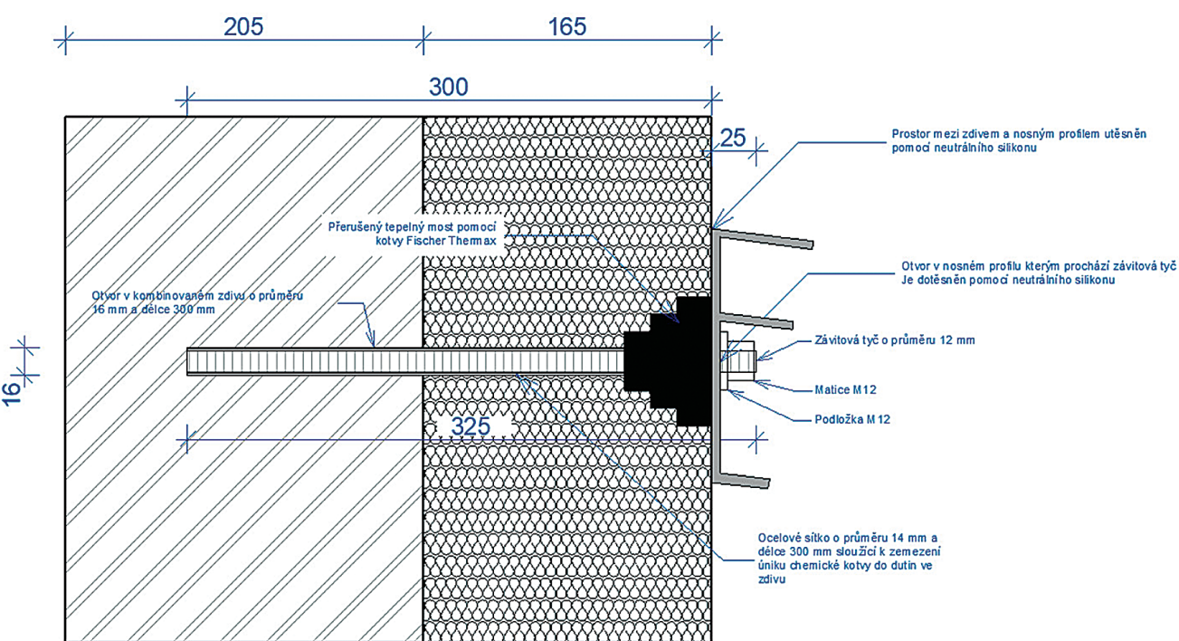
Systém s přerušeným tepelným mostem (PTM)
