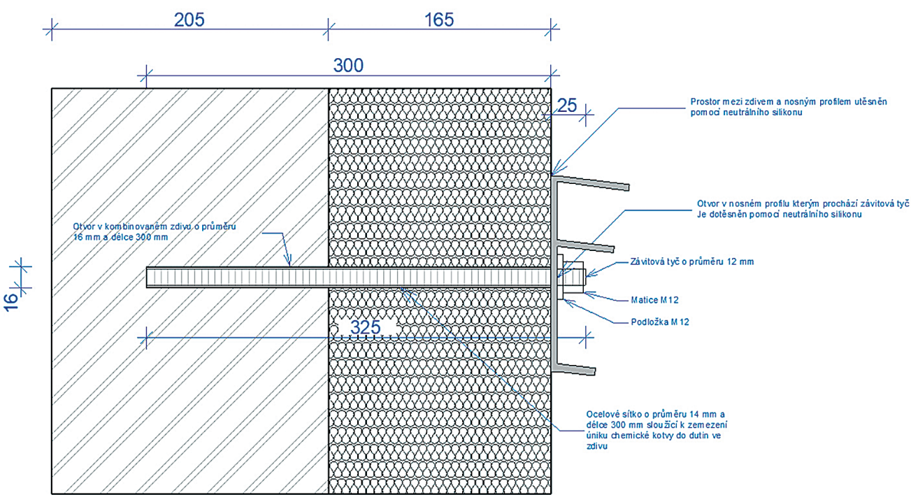
Závitová tyč
